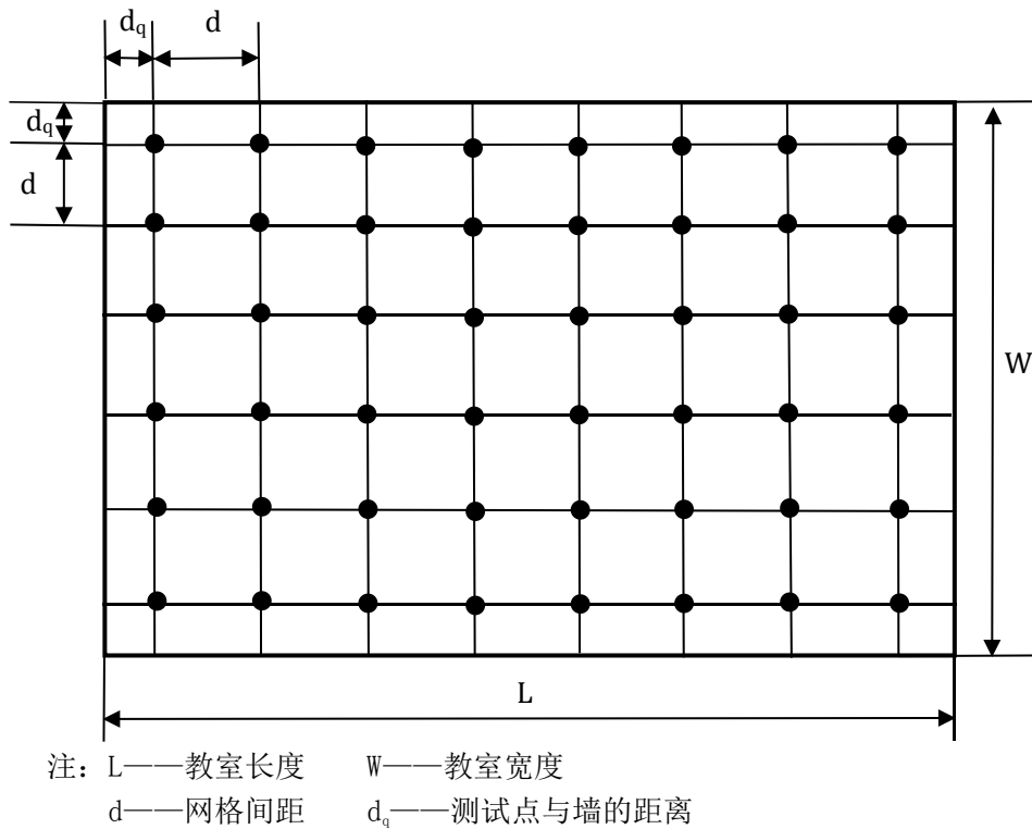
图 D3 采光点测试布点示意图
