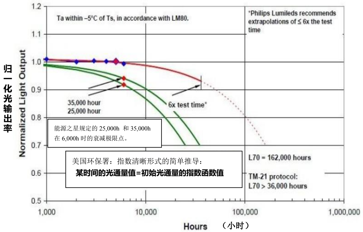
图 F1 光的衰减指数曲线
