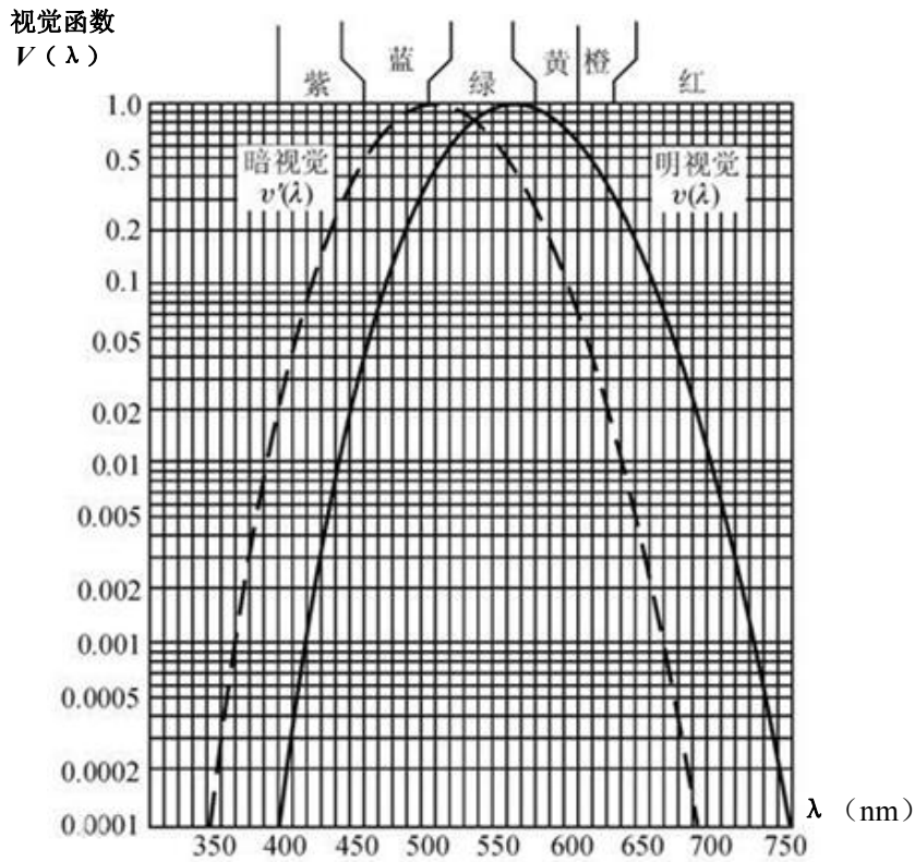
图 F3 人眼的明视觉和暗视觉函数曲线
