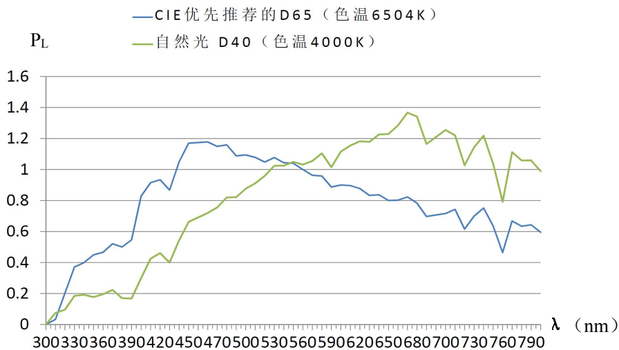
图 F1 D40 与 D65 光谱光功率分布比较
