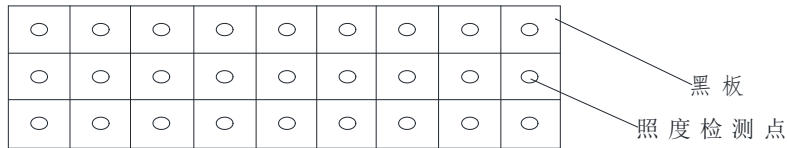
图 C2 黑板照度的测试点分布平面图
