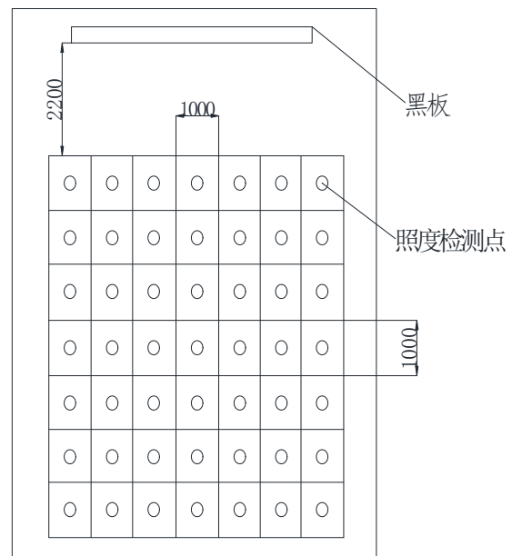
图 C1 教室照明照度的测试点分布平面图
