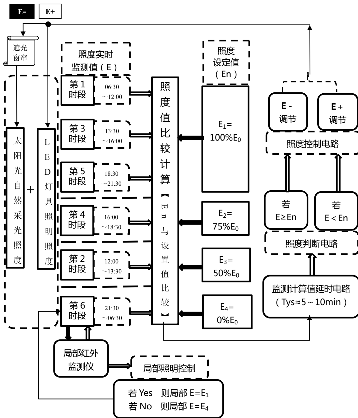
图 B2 单元教室照明智慧控制逻辑关系图
