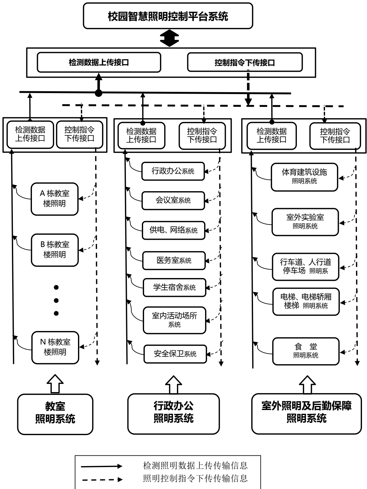
图 B1 校园照明整体智慧控制逻辑关系图
