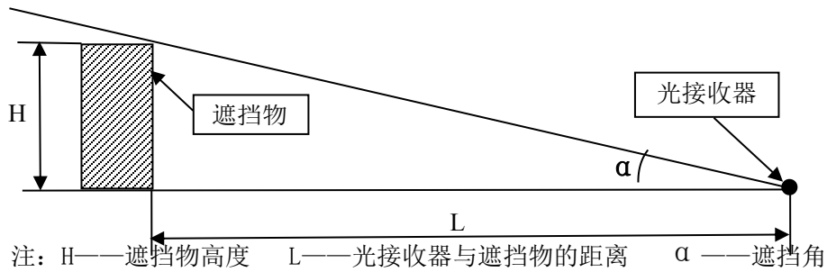
图 D2 建筑物遮挡示意图
