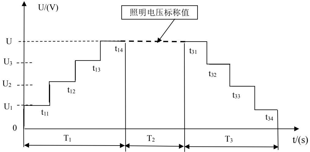
图 E3 校园智慧照明阶梯步进式软启动/软熄灭示意图
