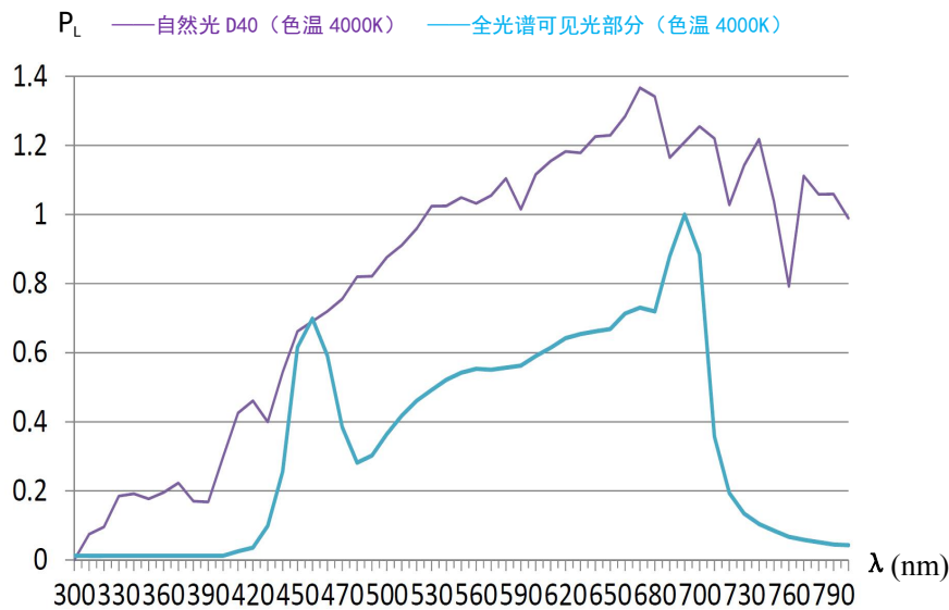
图 F2 D40 与 LED 高显指光源光源光功率分布曲线比较
