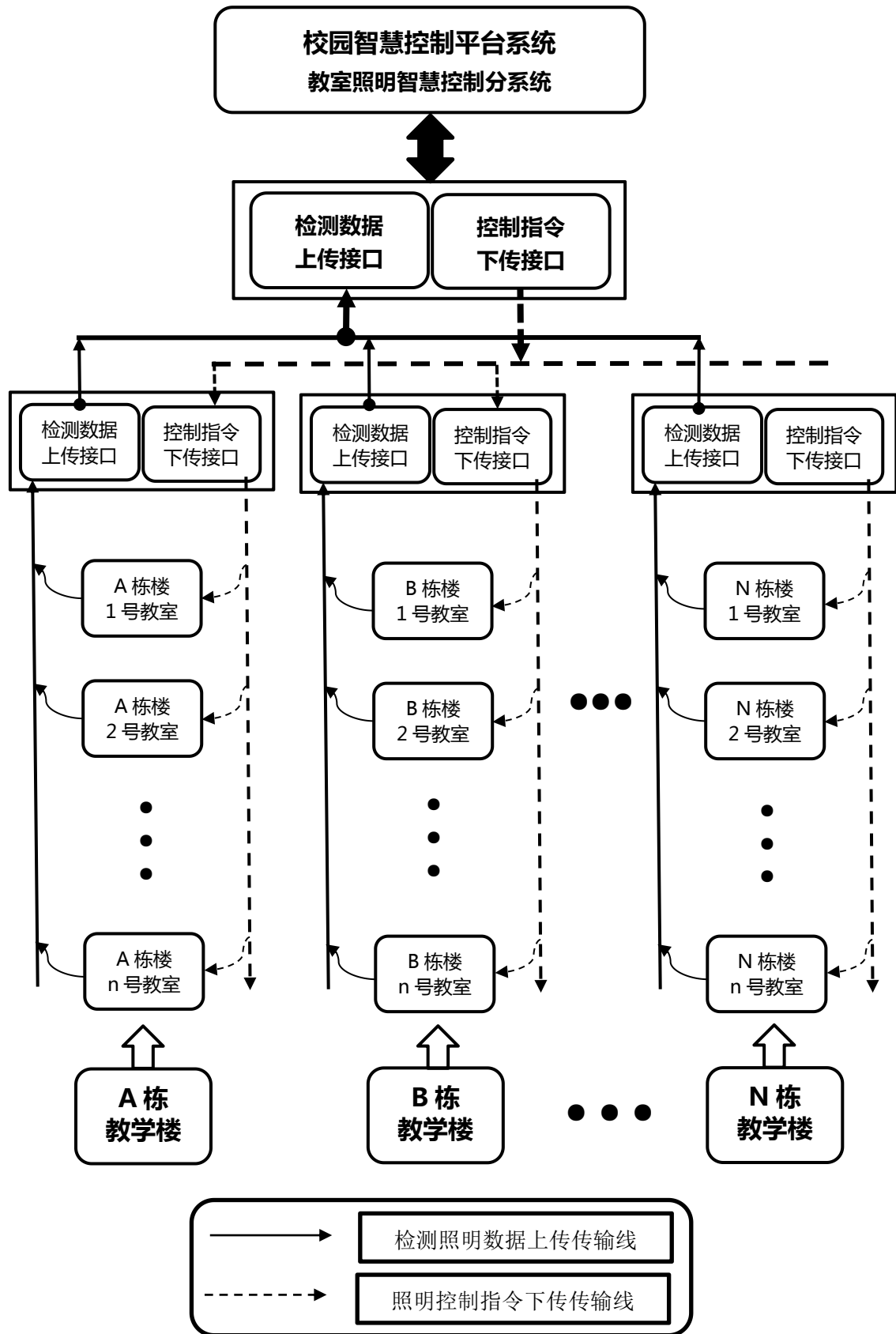
图 B3 校园教室照明系统智慧控制逻辑关系图
